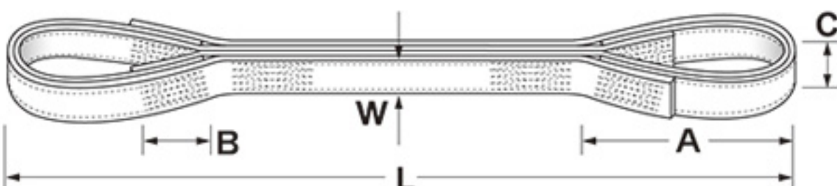
●標準仕様一覧表(WA-1)単位はmm
