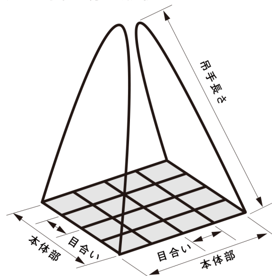
●マスク形ベルトモッコ寸法表 単位は mm
