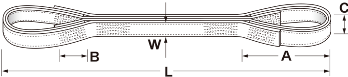
●標準仕様一覧表 (WA-1) 単位はmm
