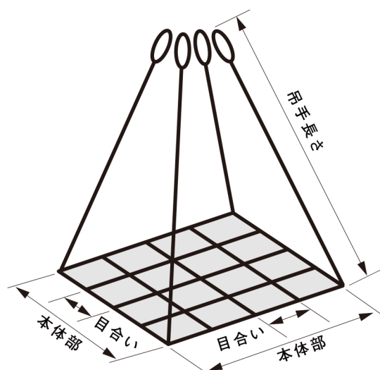
●アイ形ベルトモッコ寸法表 単位は mm
